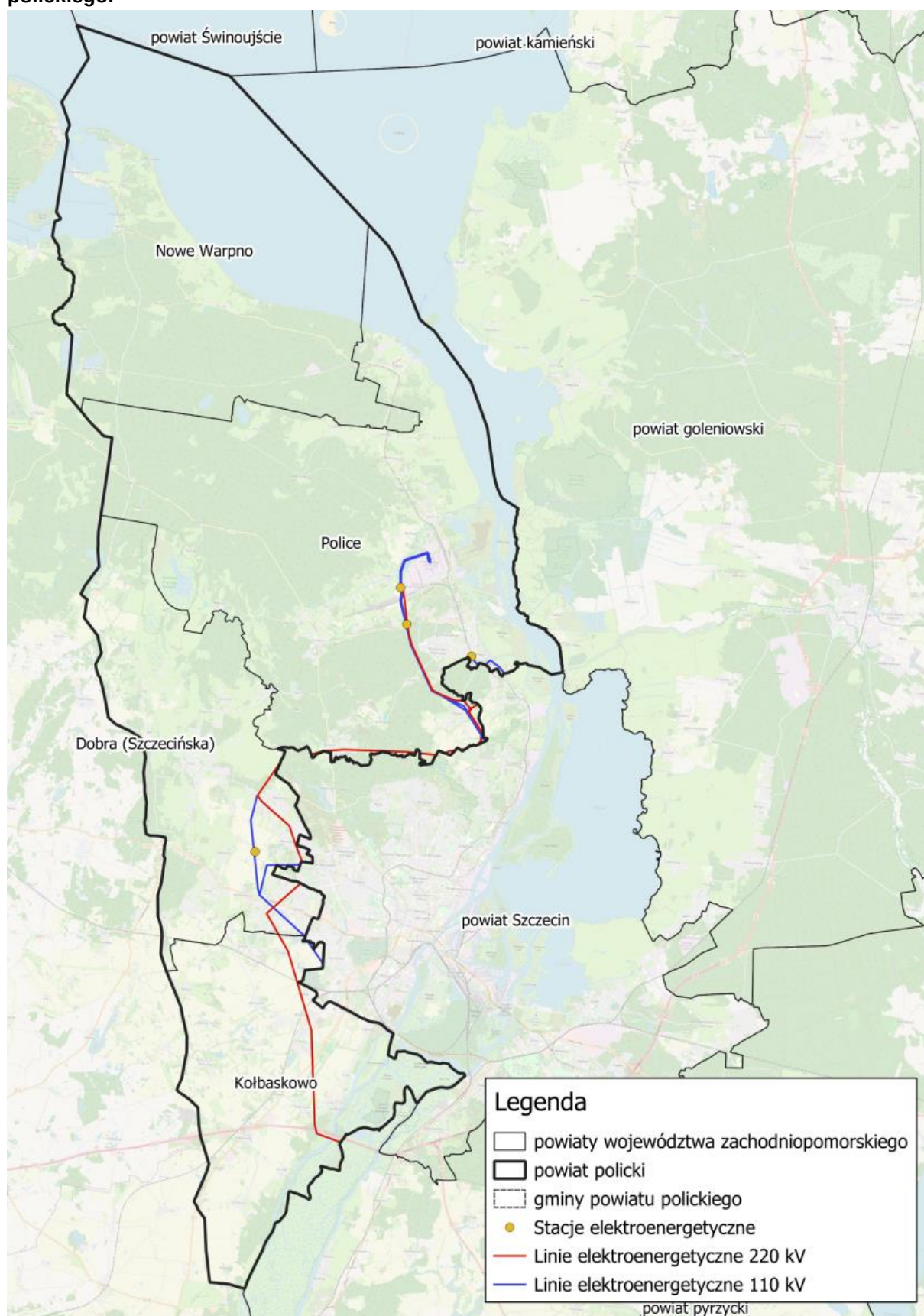
Rysunek 9. Linie oraz stacje elektroenergetyczne wysokiego napięcia, na tle powiatu polickiego.
